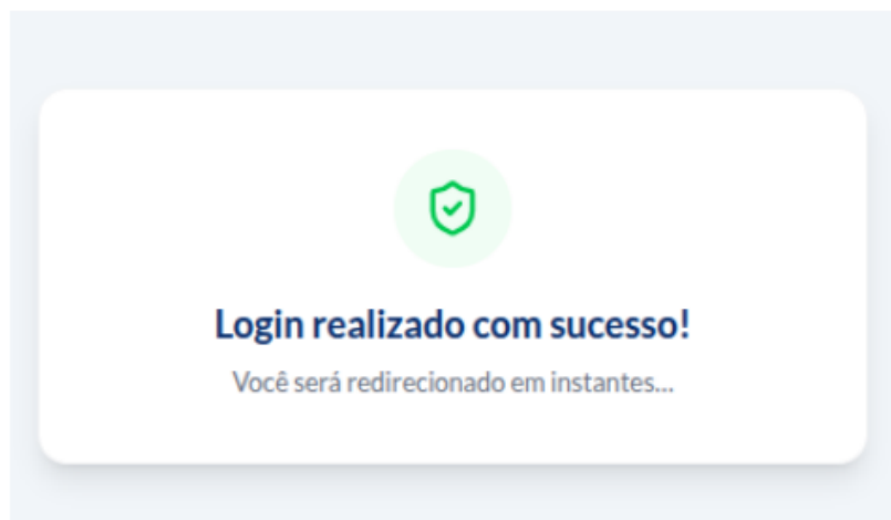
Figura 17: Login realizado
