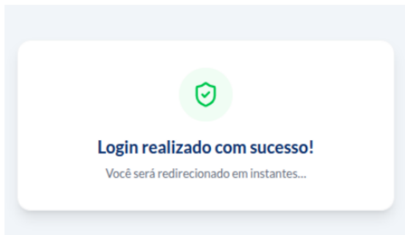
Figura 17: Login realizado
